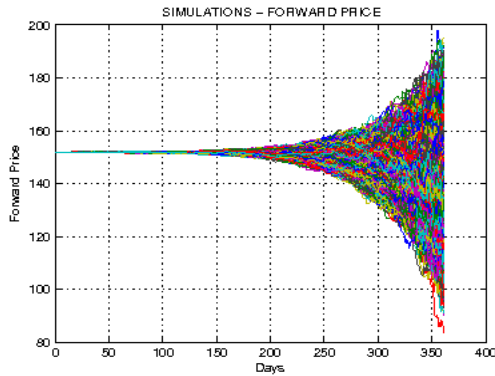
Gráfica 15. Precio forward, con Niño y con prima 10.
