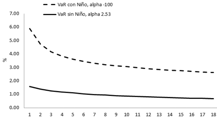
Gráfica 6. VaR para 2 días sensibilizado por prima de riesgo y vencimiento.
