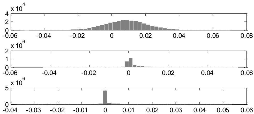
Gráfica 3. Histogramas de \psi_d^T para T = 18 meses y d = 1, 15, 30 días.
