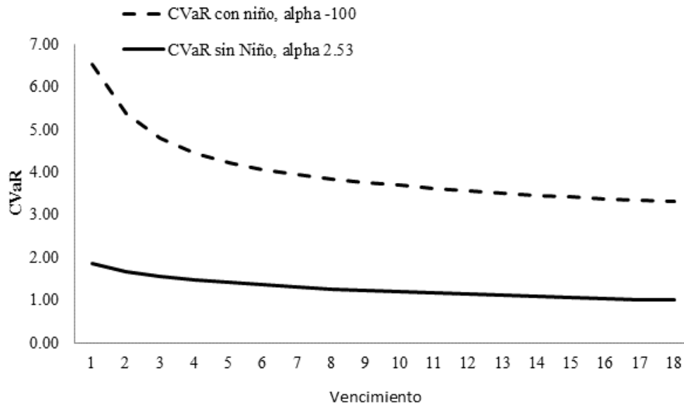
Gráfica 8.C VaR para 2 días sensibilizado por prima de riesgo y vencimiento.
